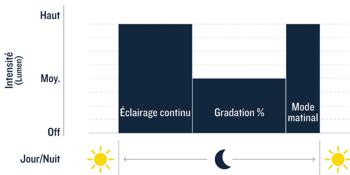
PROFIL D'OPÉRATION (SOIR 100%, GRADATION, MATIN 100%)
