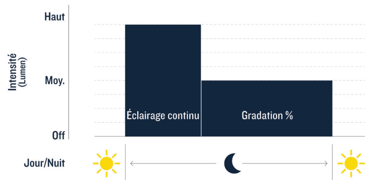
PROFIL D'OPÉRATION (SOIR 100%, ENSUITE GRADATION)
