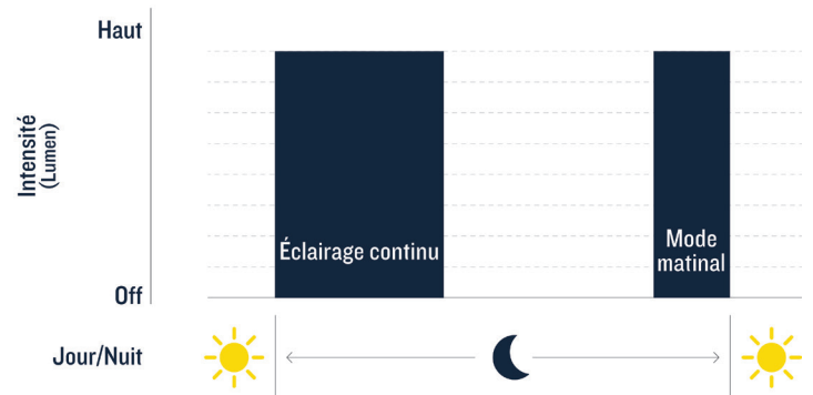
PROFIL D'OPÉRATION (SOIR 100%, OFF, MATIN 100%)
